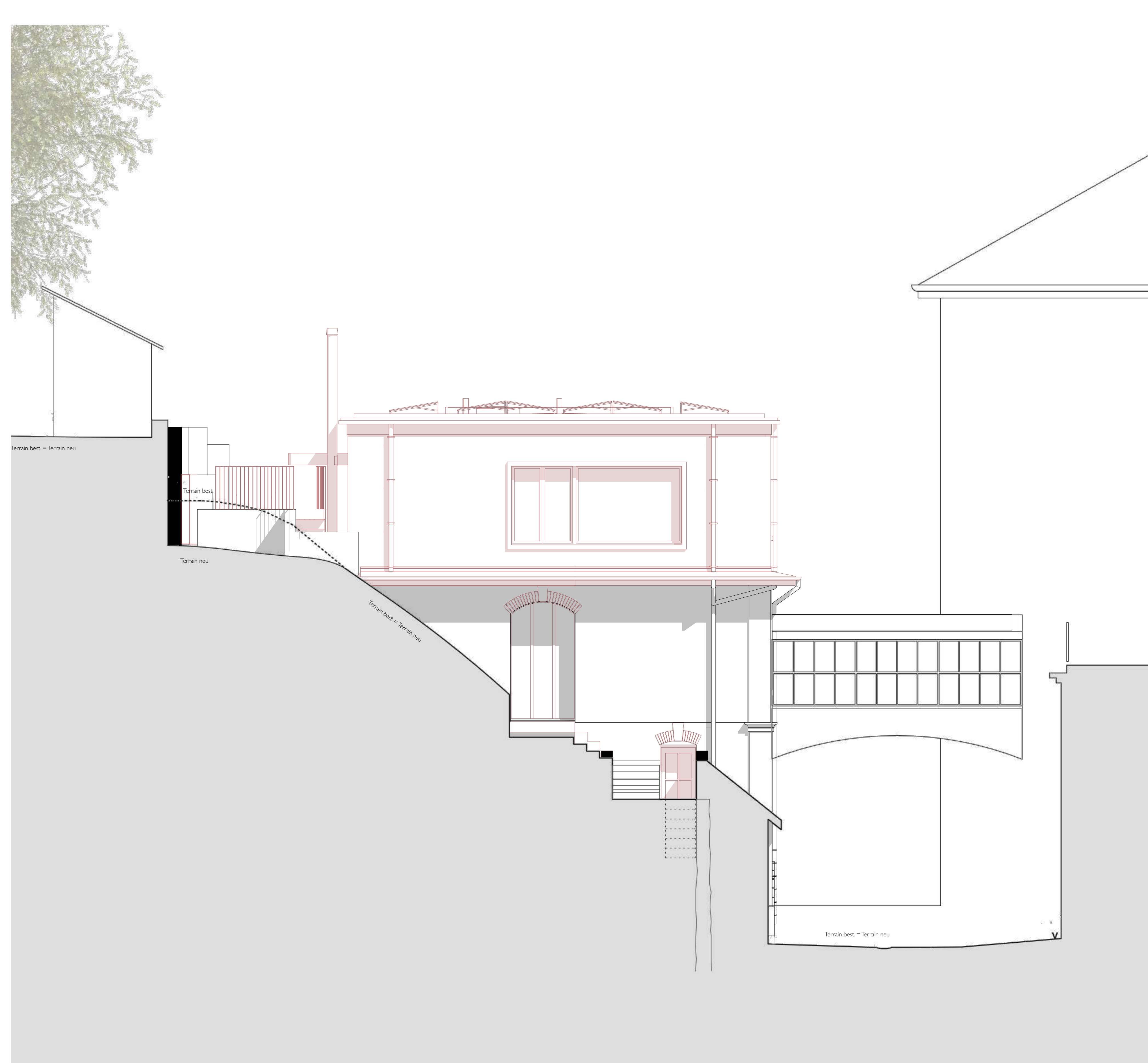
04 Nord-Ost Nord-Ost 1:50
