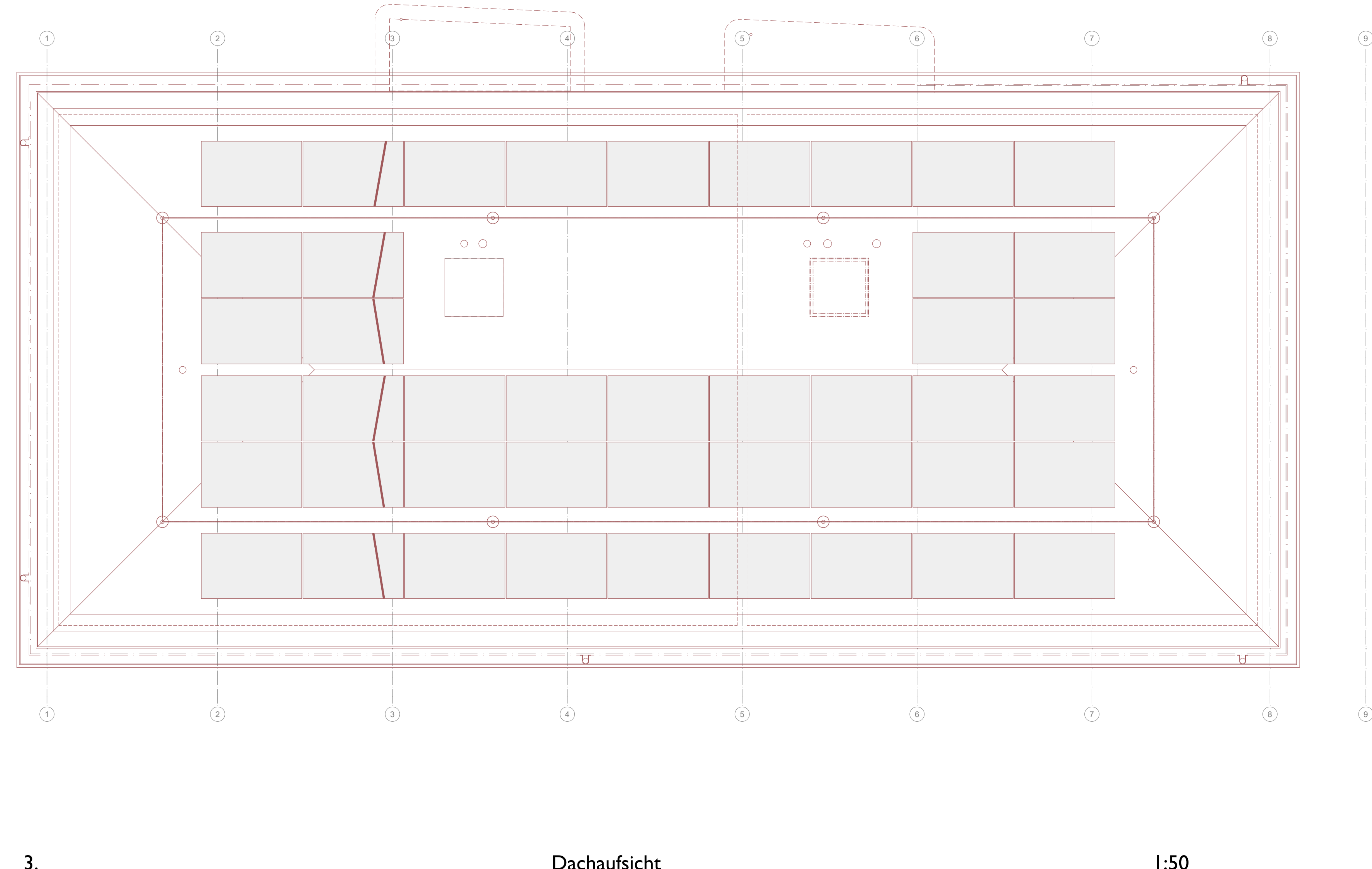
3. Dachaufsicht 1:50
