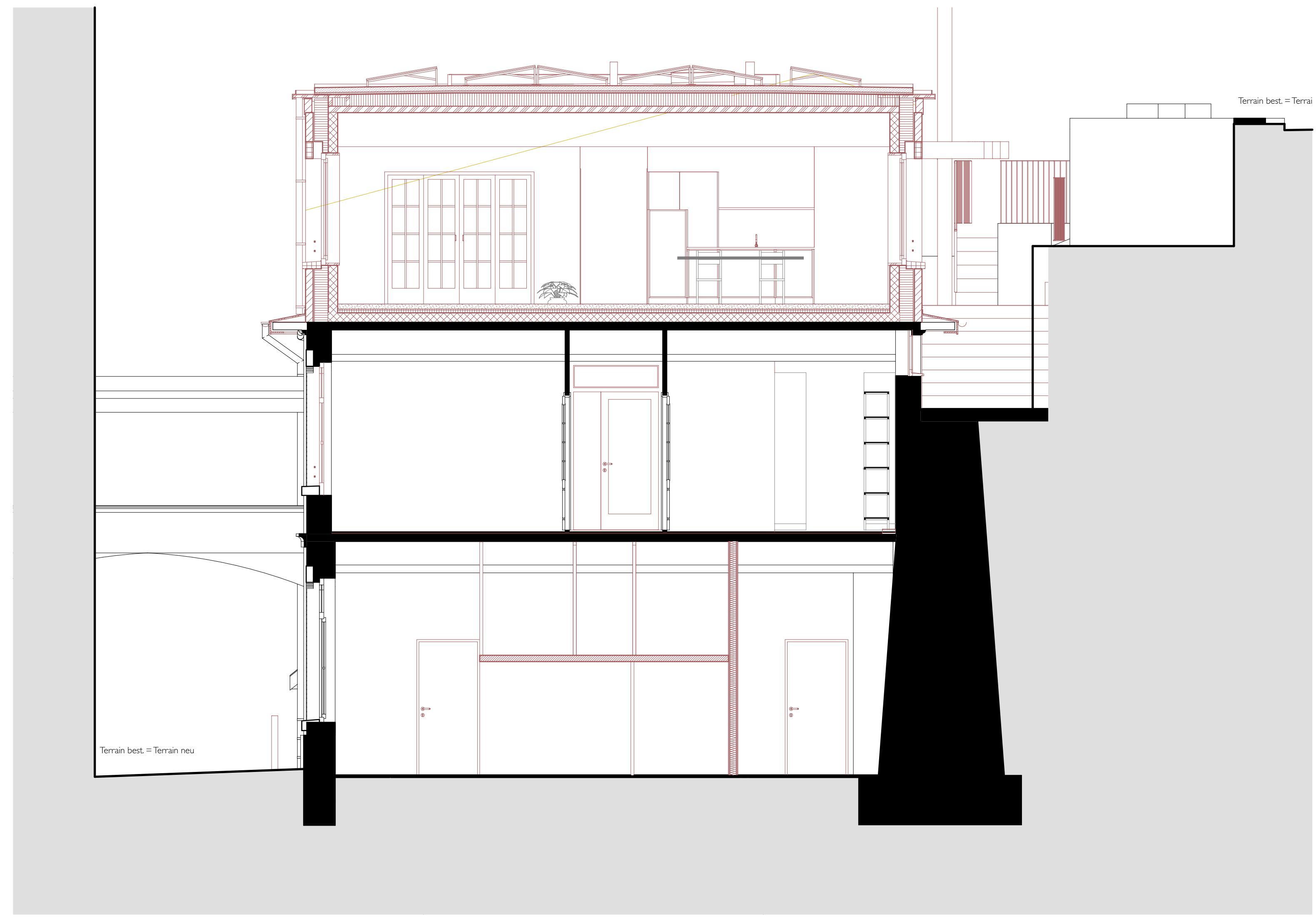
QS-A Querschnitt A 1:50
