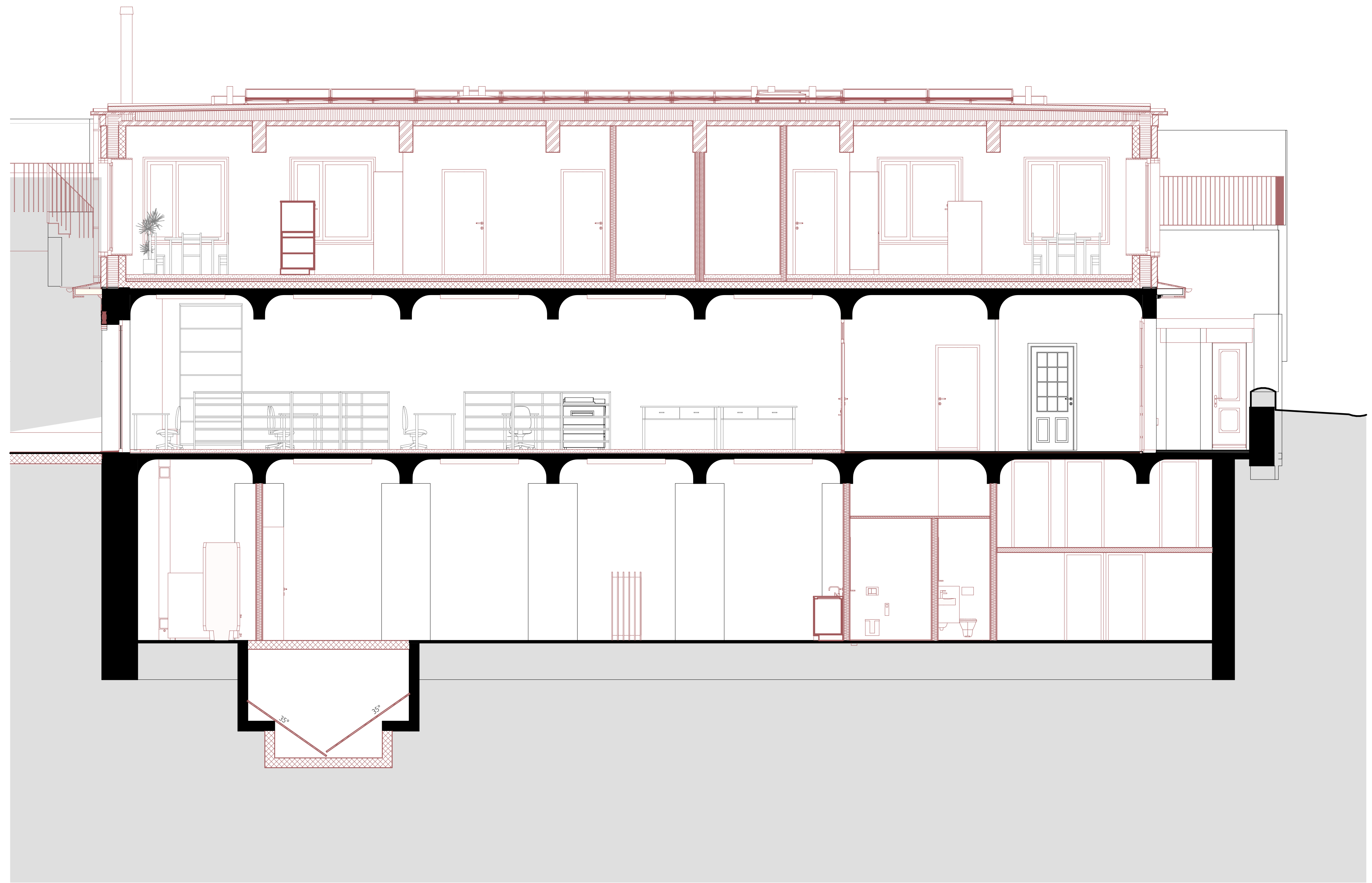
LS-C Längsschnitt C 1:50
