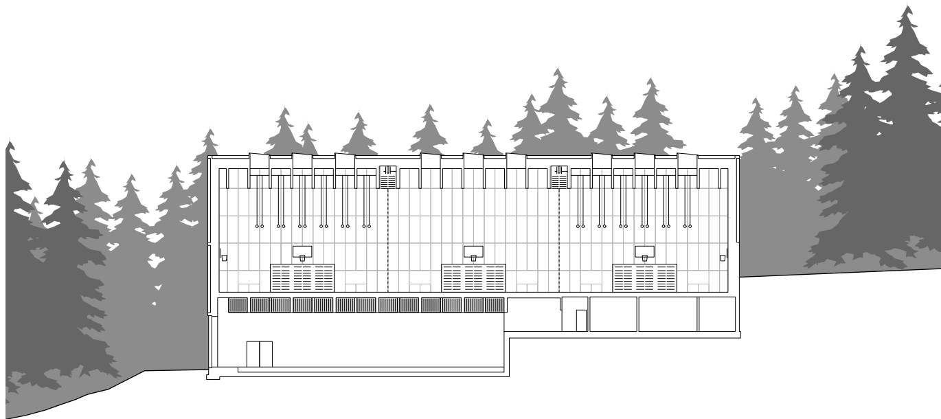
COUPE LONGITUDINALE
