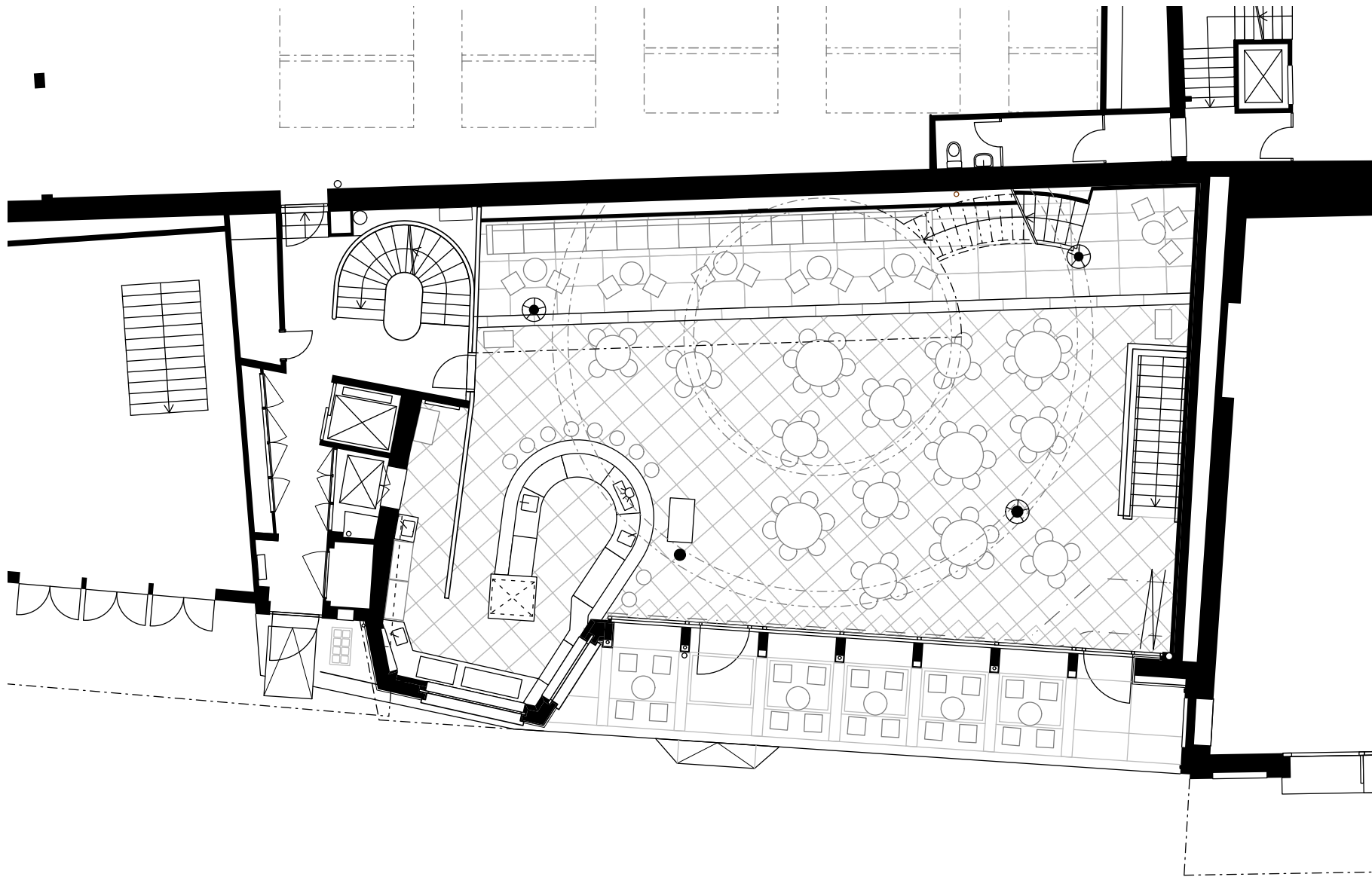
Grundriss EG 1:250
