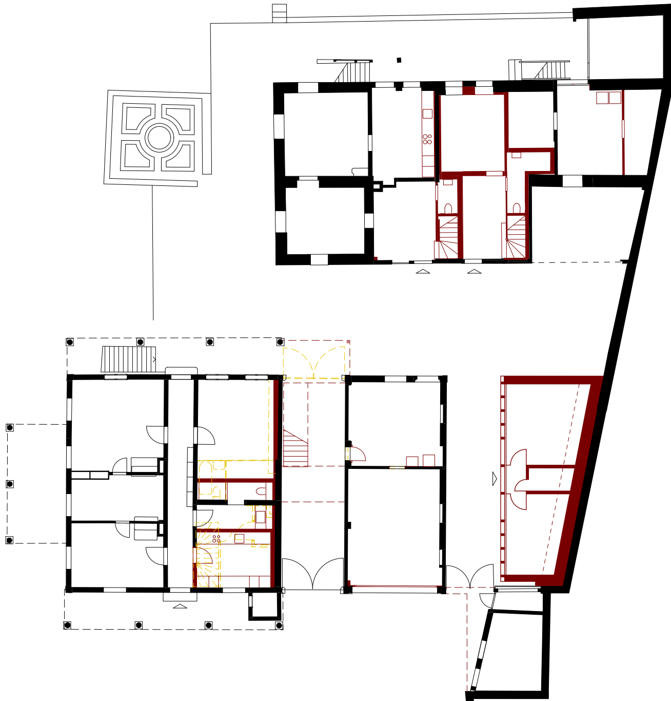
Grundriss Erdgeschoss
