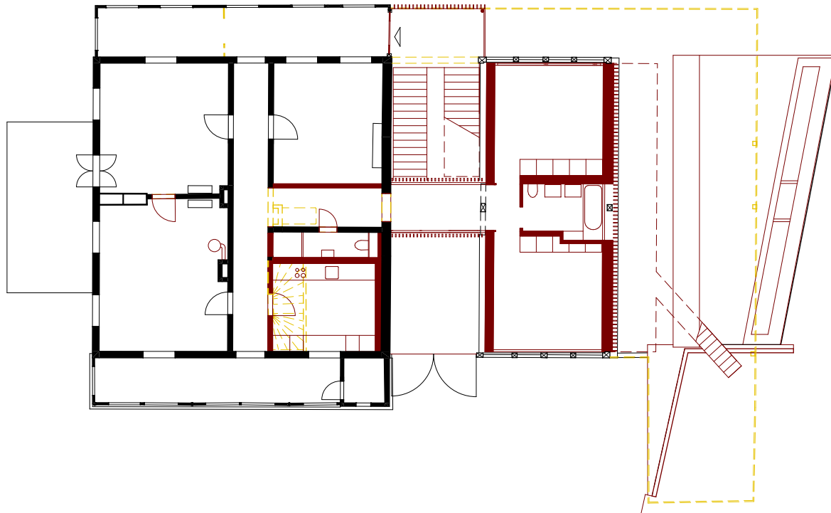
Grundriss Erdgeschoss
