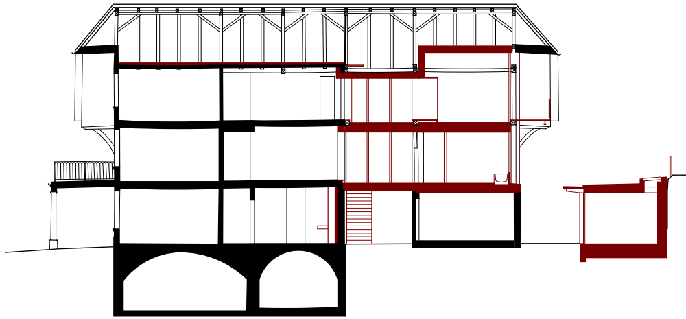
Längsschnitt Haupthaus Wohnstock mit Ökonomieteil
