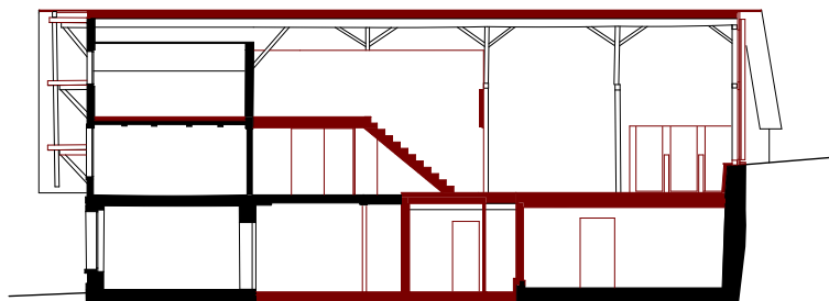
Längsschnitt Stöckli
