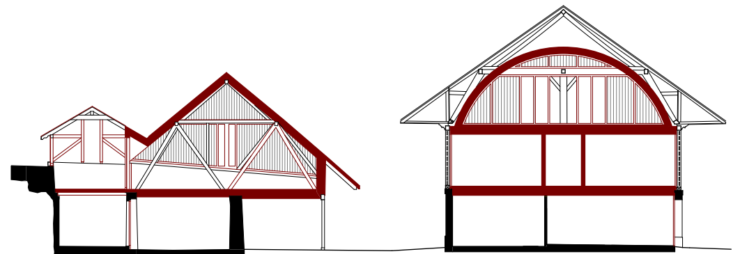
Querschnitt Stöckli und Ökonomieteil Haupthaus
